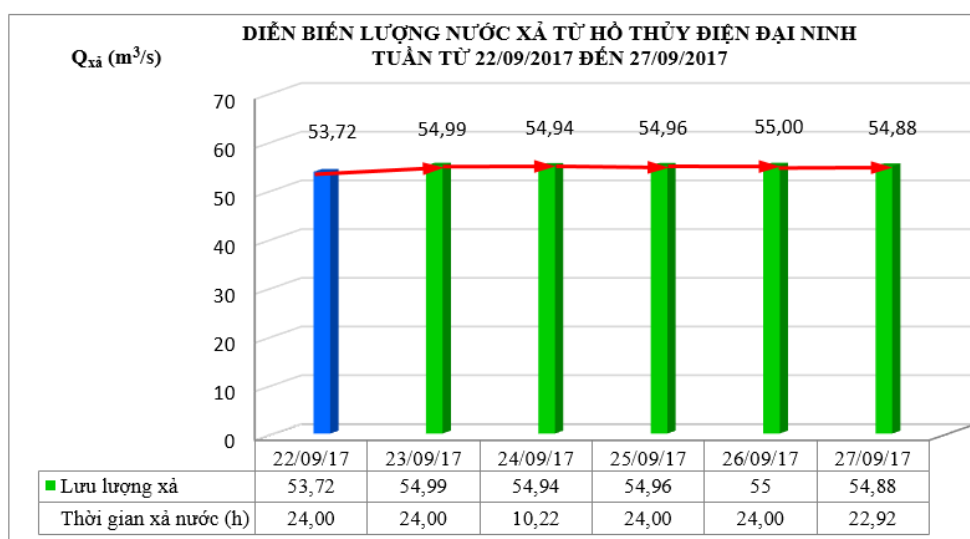
Hình 2: Diễn biến lượng nước xả từ hồ Thủy điện Đại Ninh từ ngày 22/09/2017 đến 27/09/2017
