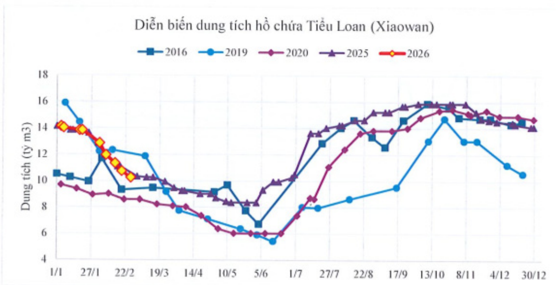
Hình 5: Dung tích trữ của hồ Tiểu Loan một số năm
